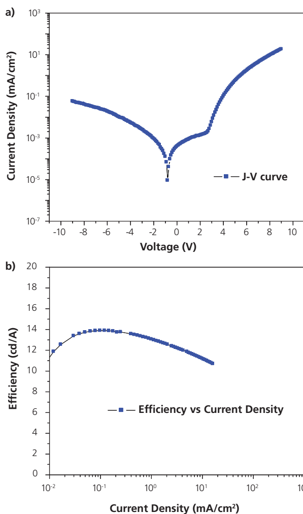
図 9. 図 8 の構造を持った緑色燐光有機 EL の (a) J-V 特性 (b) 電流効率 - 電流密度のグラフ
