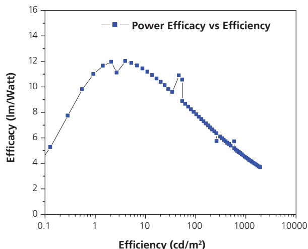
図10. Plexcore® OC を正孔注入層として使用した燐光有機 EL 素子の発光効率。図に見られるとおり、発光効率のロスは輝度が 1000cd/m² まで最小限に抑えられています。
