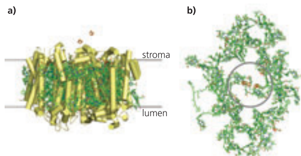
図 2. a) PS I の膜内 \alpha -らせん (黄色の管) は、アンテナ Chl a 分子 (緑色) と反応中心近傍の電子伝達補因子に対する骨格として機能します。[4Fe-4S] クラスター ( F_A と F_B ) がストロマ側に見えています。b) 図 a) を 180^\circ 回転してタンパク質骨格を取り除いてストロマ側から見ると、反応中心近傍の電子伝達補因子 (グレーの円内) の周囲にあるアンテナ Chl a 分子の組織を見ることができます。
