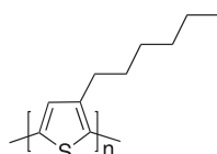
図 1. ポリ 3-ヘキシルチオフェンの構造
