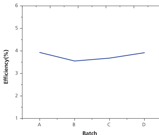
図 4. Plexcore ® OS 2100 を用いて作製した P3HT:PCBM 系有機太陽電池の効率に関するバッチ間データ
