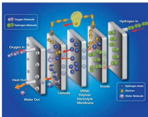
図1. 水素燃料と空気中の酸素で動作する高分子電解質膜燃料電池の模式図
