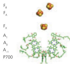
図 3. 反応中心近傍の電子伝達補因子は、光誘起により電子が P700 から補因子を通して F_B に高速に移動するように配置されています。まず、P700 と A_0 の間に電荷分離状態が確立されます。次に、電子が A_1 (結合フィロキノン分子) に、続いて 3 つの [4Fe-4S] クラスターに移動します。3 つのうち、最初のクラスターであるポリペプチド間 [4Fe-4S] クラスター ( F_x ) は、PsaA と PsaB の両方が供給するシステイン残基とライゲート (ligate) しています。ストロマ側の PsaC タンパク質は、2 つの末端 [4Fe-4S] クラスター ( F_A と F_B ) を支持しています。
