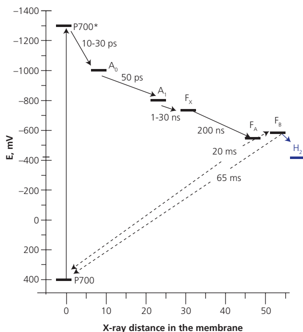
図 4. 電子が P700 から離れるにつれて補因子の電位が高くなるため、熱力学的に有利になります。水素発生の酸化還元電位は F_B クラスターより高い電位のため、 F_B^- から H_2 発生部位（Pt ナノ粒子またはヒドロゲナーゼ酵素）へのさらなる電子移動も熱力学的に有利です。
