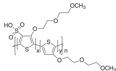
図 7. スルホン化ポリ (チオフェン-3-[2-(2-メトキシエトキシ)エトキシ]-2,5-ジイル) の構造
