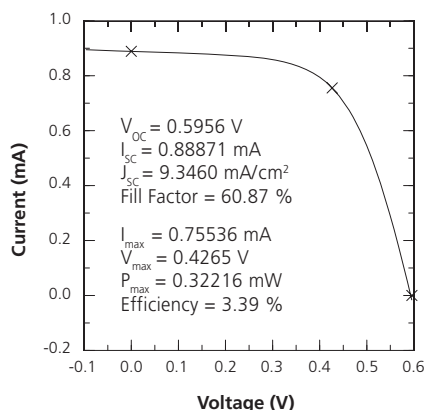
図 6. NREL が認定した Plexcore® OS 2100:PCBM 有機太陽電池の電流 - 電圧曲線。(デバイス温度: 27.0 ± 3.0°C、デバイス面積: 0.095 cm²、放射照度: 1000.0 W/m²)
