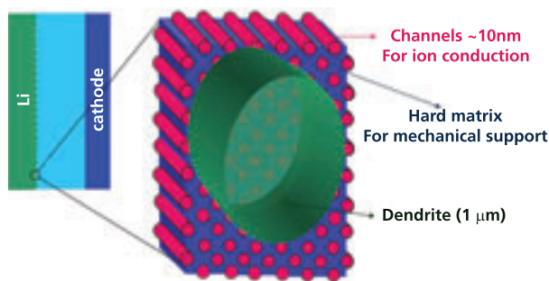
図 3. 新規複合体電解質を用いた電池の模式図
